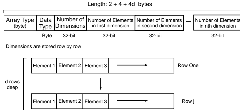
FIG. 7. Array data type.
